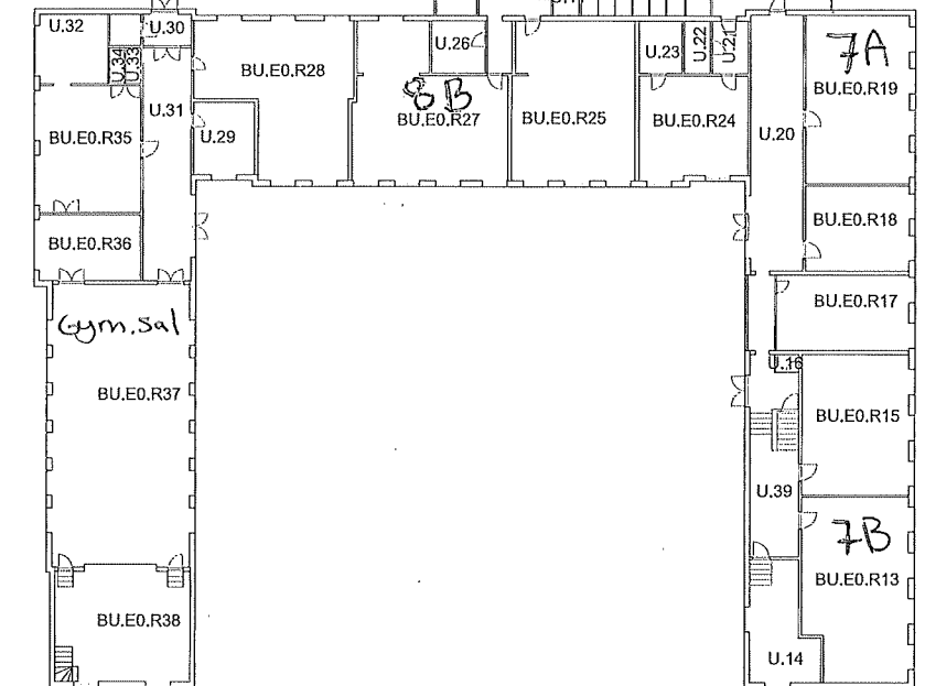
Byg U Stueplan
