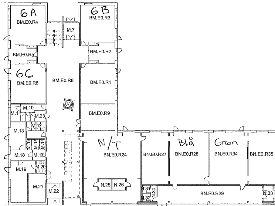
Stueplan Byg M
