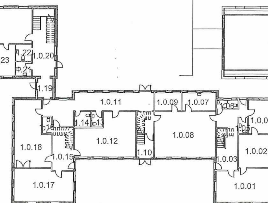
SFO - Stueplan
